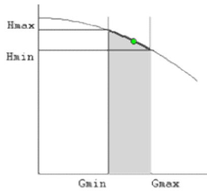
Рисунок 5. Напорно-расходная характеристика насоса
