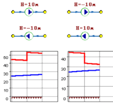
Рисунок 4. Пьезометрические графики
